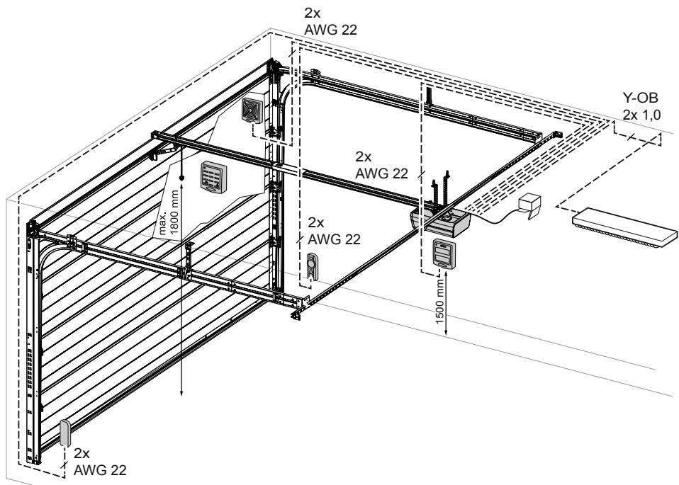
Abb. 3: Beispielininstallation Zubehör
