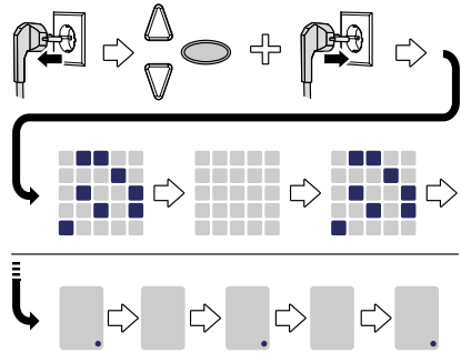
Abb. 6: Löschen aller am Antrieb programmierten Handsender
