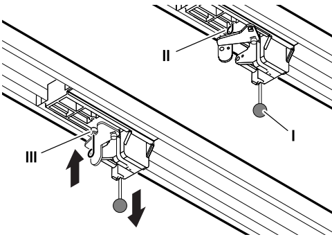
Abb. 9: Antrieb entriegeln und verriegeln
