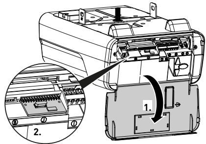
Abb. 10: Abdeckung des Antriebskopfes öffnen und Funkmodul bestimmen
