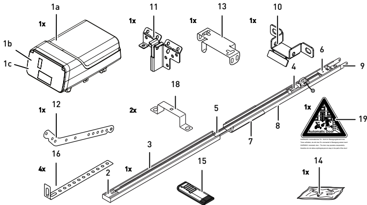
Abb. 2: Produktübersicht - Einzelteile
