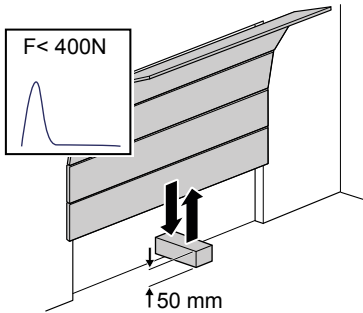
Abb. 7: Kraftbegrenzung prüfen
