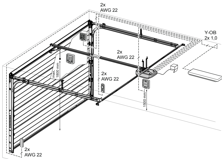
Afb. 3: Voorbeeldinstallatie accessoires
