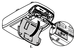
Fig. 10: Aprire il coperchio della testa motrice e definire il modulo radio
