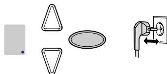
Fig. 6: Eliminazione di tutti i trasmettitori portatili programmati sul motore
