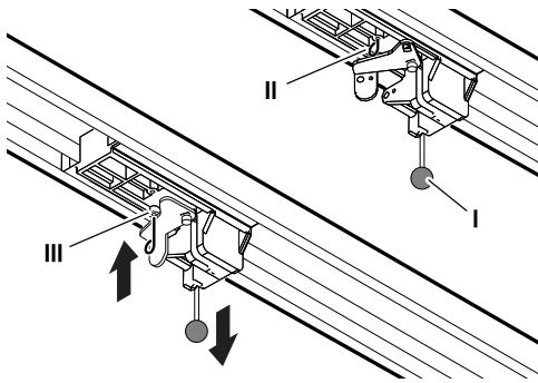
Fig. 9: Sbloccaggio e bloccaggio del motore
