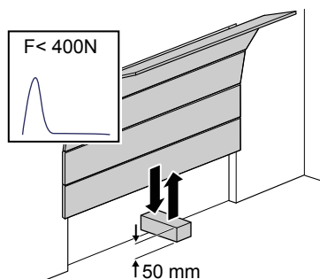
Fig. 7: Contrôle de la limitation d'effort
