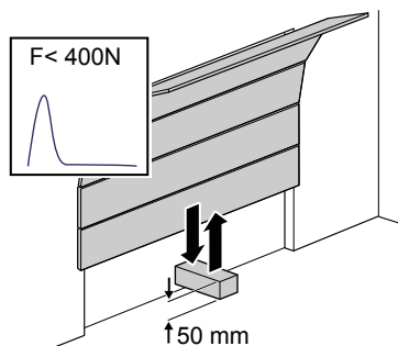
Fig. 7: Kontrollere kraftbegrensningen
