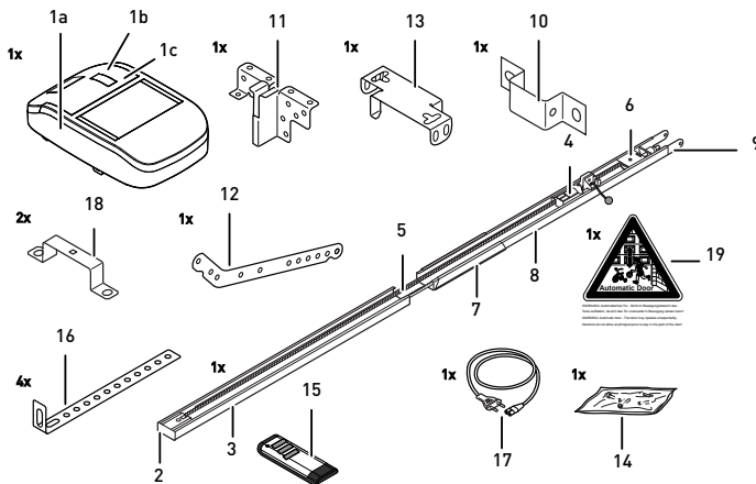
Fig. 2: Produktoversikt - Enkeltdele
