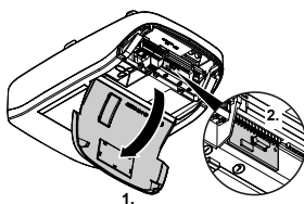
Abb. 10: Otvaranje poklopca pogonske glave i određivanje radijskog modula
