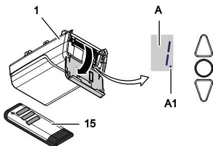
Fig. 4: Éléments de commande
