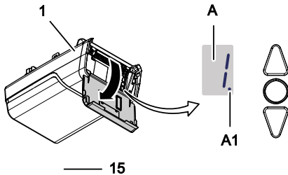
Abb. 4: Bedienelemente
