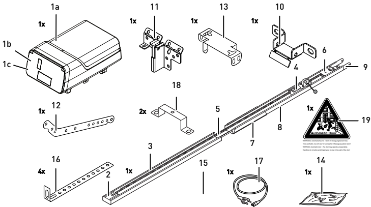
Abb. 2: Produktübersicht - Einzelteile
