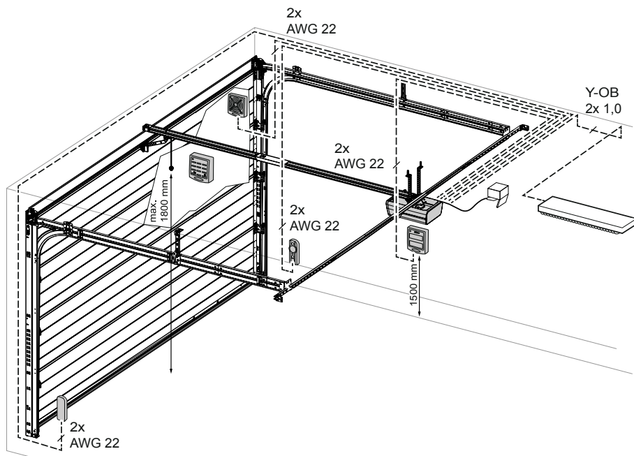
Rys. 3: Instalacja przykładowa wyposażenia dodatkowego
