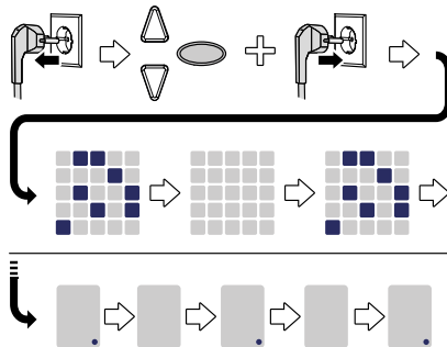
Rys. 6: Usuwanie z pamięci wszystkich nadajników ręcznych zaprogramowanych w napędzie
