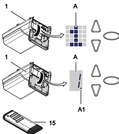
Rys. 4: Elementy sterowania oraz wersje wyświetlacza cyfrowego
