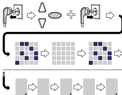
Fig. 6: Slette alle håndsendere som er programmert på drevet
