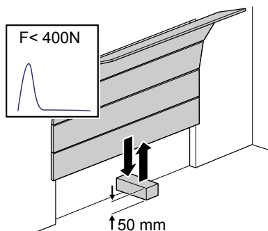
Fig. 7: Kontrollere kraftbegrensningen
