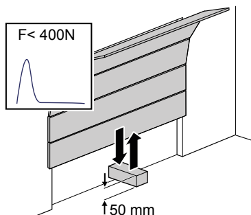
Afb. 7: Krachtbegrenzing controleren
