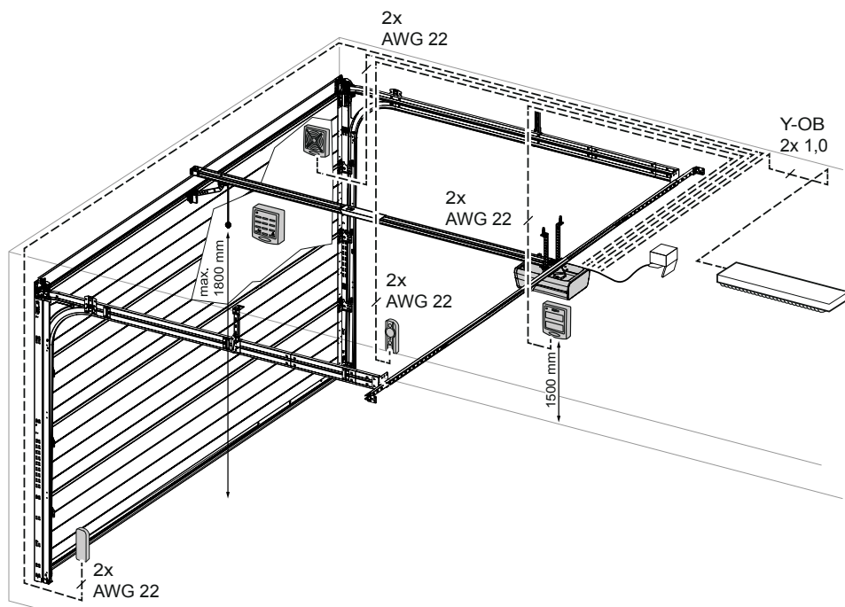
Afb. 3: Voorbeeldinstallatie accessoires
