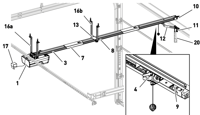
Afb. 1: Productoverzicht - opgebouwd
