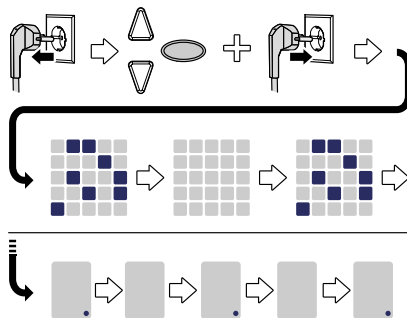
Fig. 6: Eliminazione di tutti i trasmettitori portatili programmati sul motore
