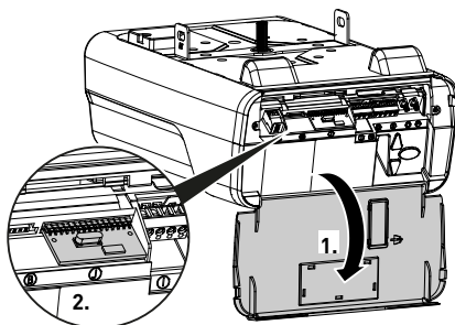
Fig. 10: Aprire il coperchio della testa motrice e definire il modulo radio
