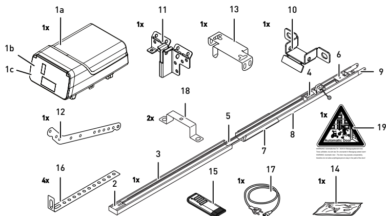
Fig. 2: Panoramica prodotto - singole parti
