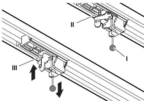
Fig. 9: Sbloccaggio e bloccaggio del motore
