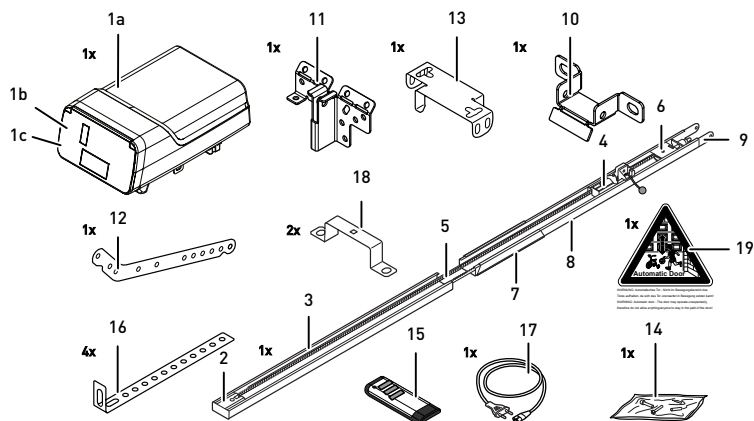
Fig. 2: Produktoversigt - enkeltdele
